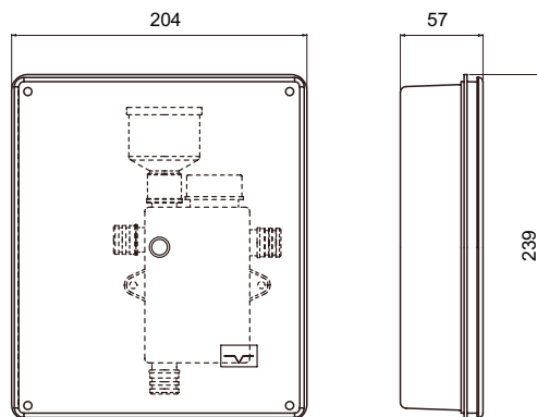
Szerelődoboz a szifonnal Box with trap
