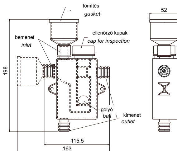
Szerelődoboz a szifonnal Box with trap
